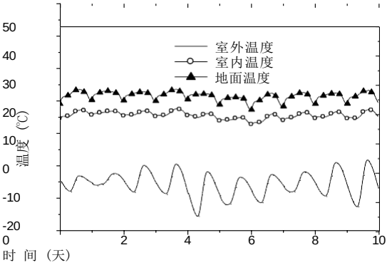
图 3 相变蓄能地板采暖效果图
