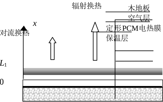
图 2 相变蓄能电采暖地板结构图
