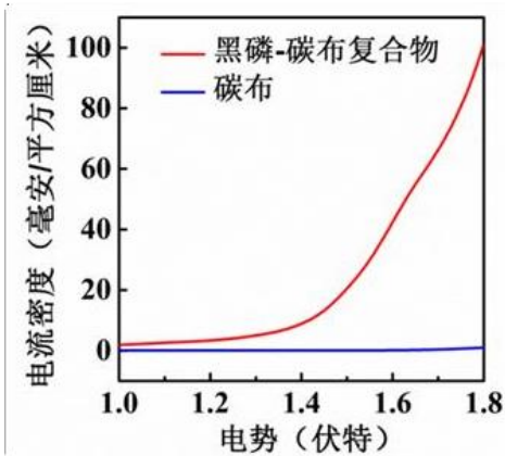
图 2 电化学析氧反应特性
