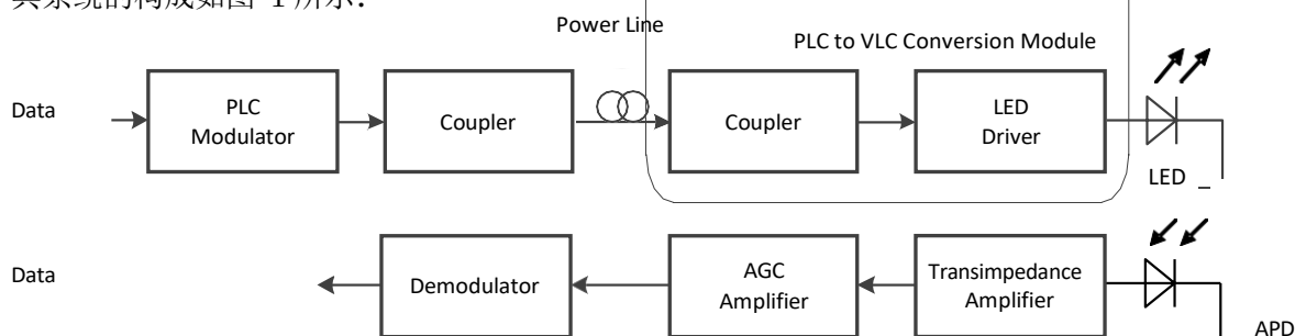
图 1 PLC+VLC 系统框图
