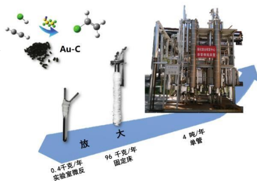
图 1 催化剂逐级放大过程
